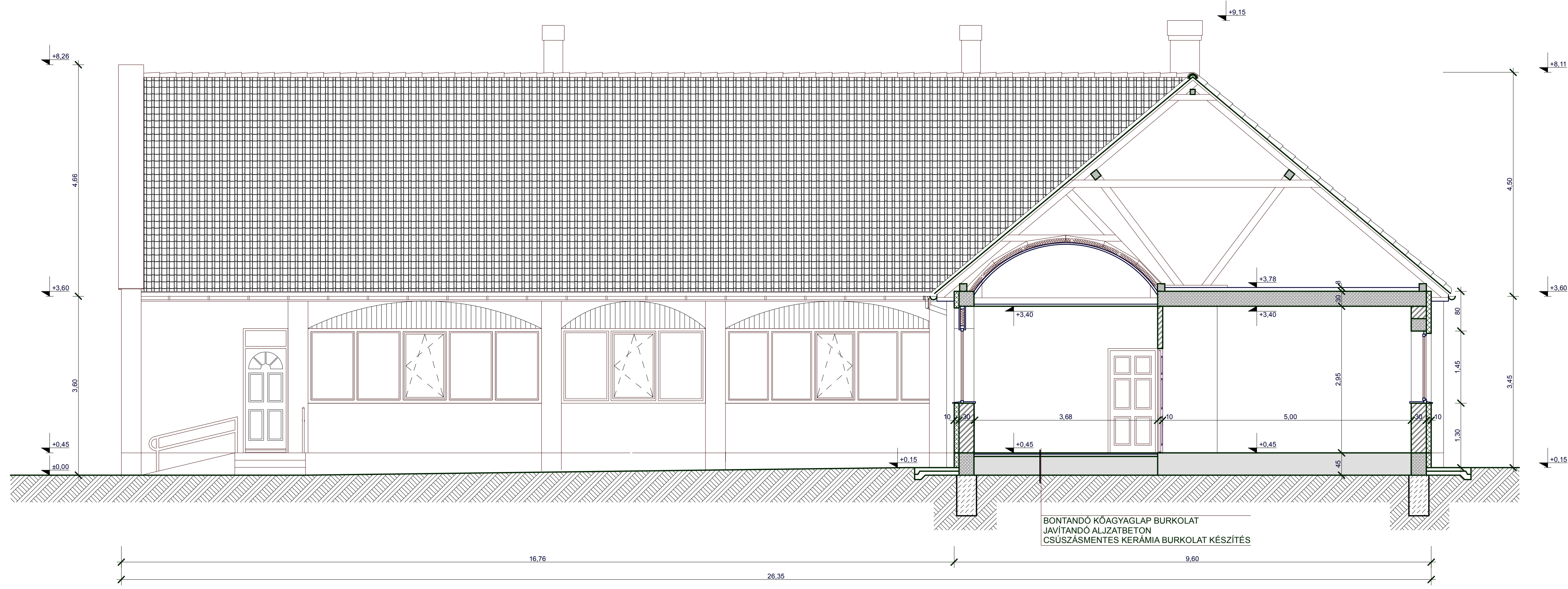
B - B METSZET
